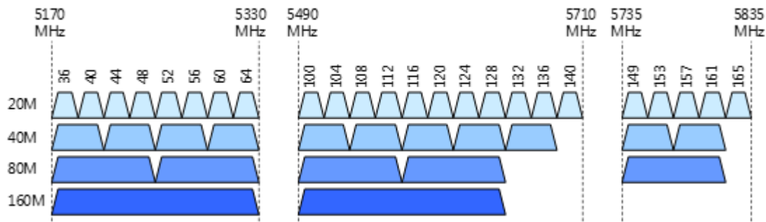
图1-5 Wi-Fi 5G 频段的信道
