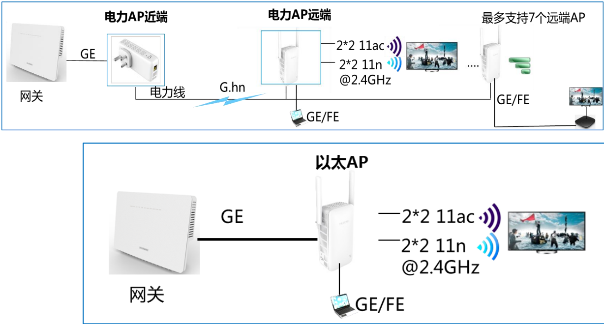
图5-2 电力/以太/Wi-Fi AP 扩展 Wi-Fi 示意图
